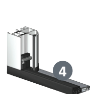
Seuil et joint cornière
