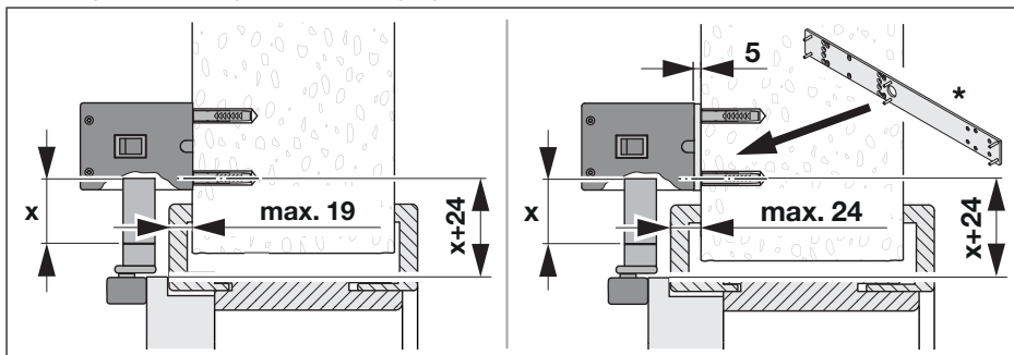
Montage aandrijving met asverlenging
