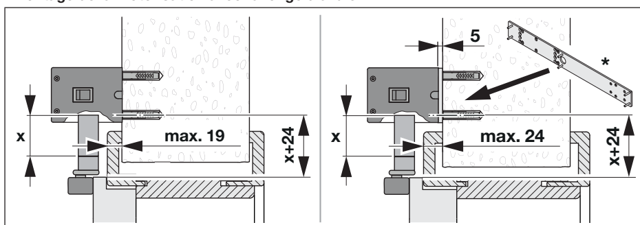
Montage de la motorisation avec rallonge d'arbre
