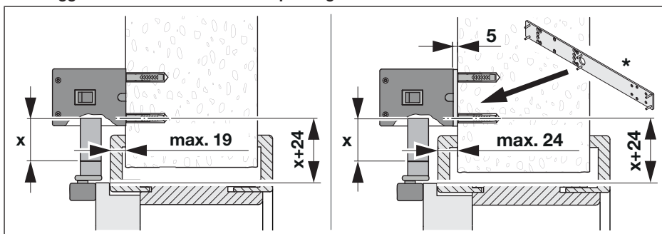
Montaggio della motorizzazione con prolunga alberi
