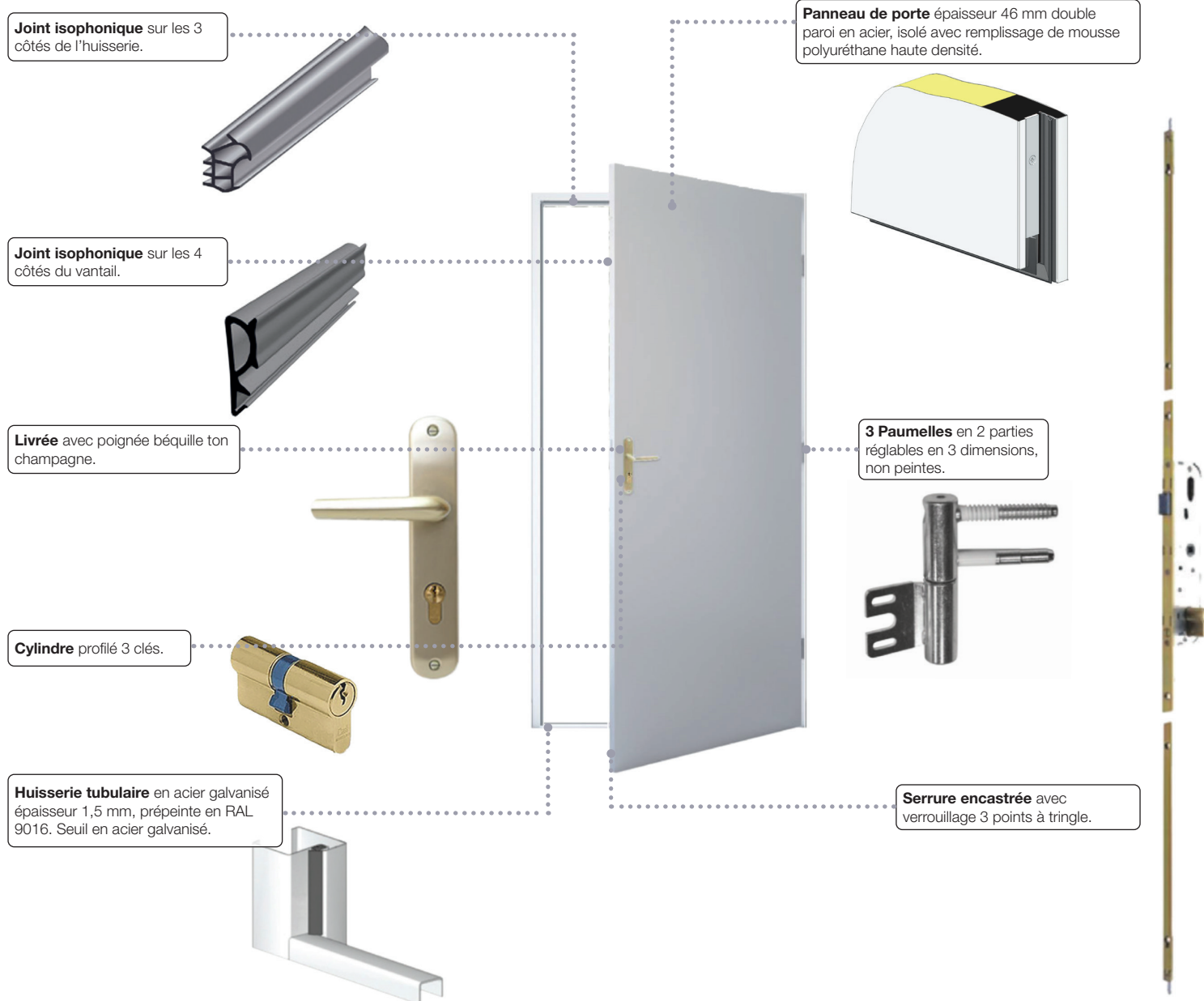
Profil d'huissierie
