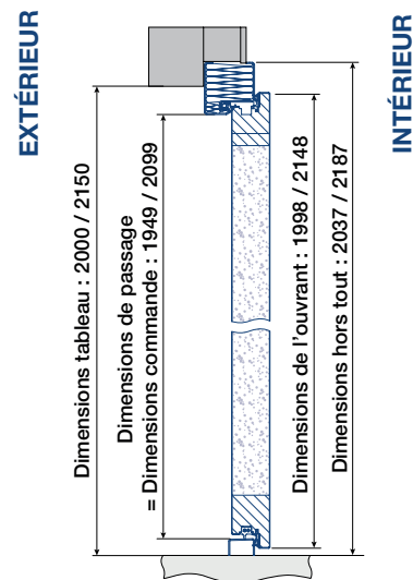
Coupe en hauteur
