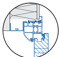
Huisserie avec tapée 100, 140 et 160 mm
