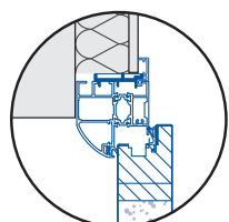
Huisserie sans tapée 60 mm
