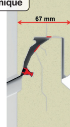
Panneaux à rupture de pont thermique
