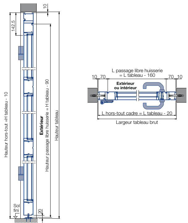
Montage dans la baie
