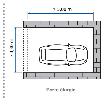
Porte standard et Bloc-porte associé
