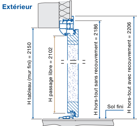
Huisserie sans tapée 60 mm
