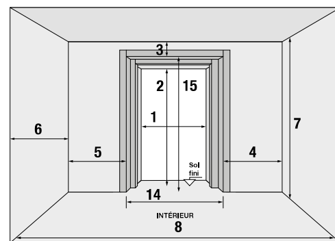
Pose avec conservation de l'ancien dormant
