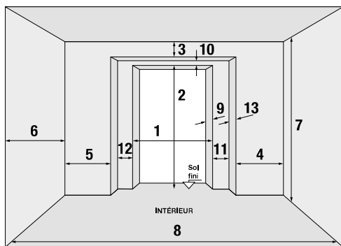
Pose en feuillure de maçonnerie après dépose totale
