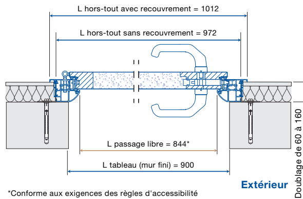
COUPE EN LARGEUR
