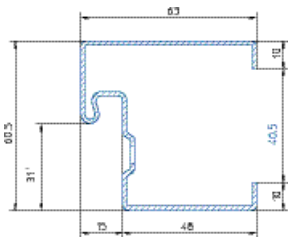
PROFIL HUISSERIE
