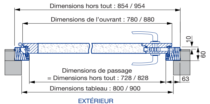
COUPE EN LARGEUR INTÉRIEUR
