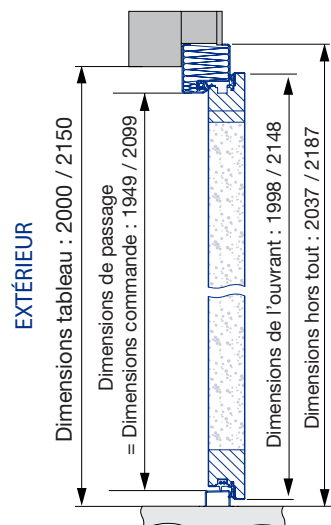
COUPE EN HAUTEUR
