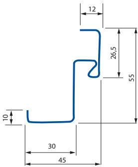
PROFIL HUISSERIE
