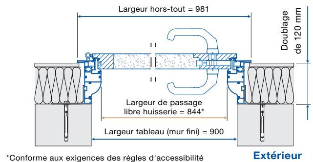
COUPE EN LARGEUR
