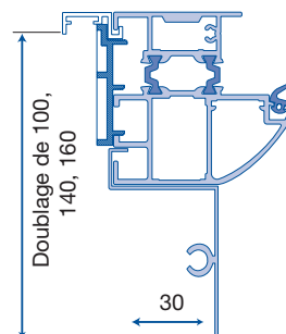
HUISSERIE AVEC TAPÉES derrière la baie
