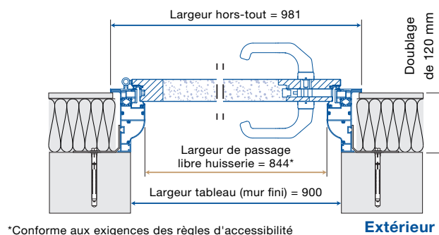
COUPE EN LARGEUR
