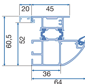
HUISSERIE SANS TAPÉES derrière la baie
