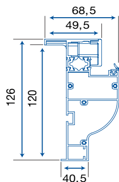
HUISSERIE MONOBLOC derrière la baie
