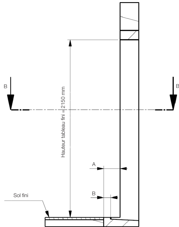
COUPE A-A
