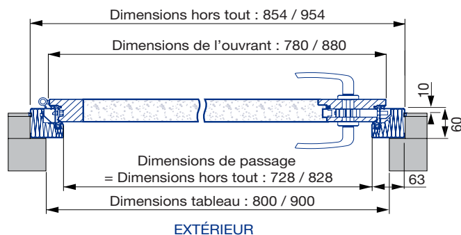
INTÉRIEUR
