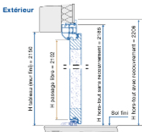
COUPE EN HAUTEUR
