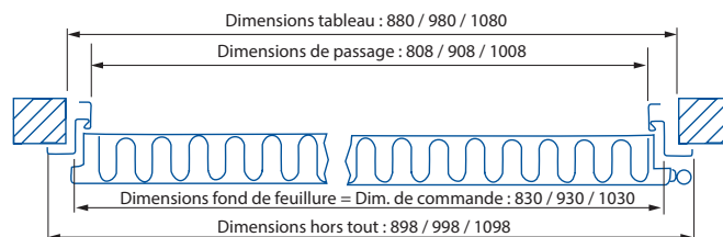
COUPE EN LARGEUR
