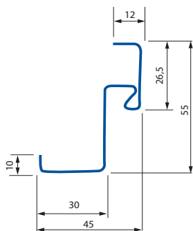
PROFIL HUISSERIE
