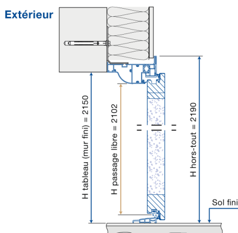
COUPE EN HAUTEUR
