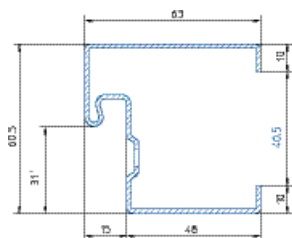
PROFIL HUISSERIE
