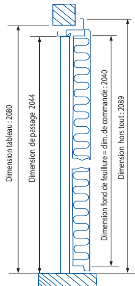
COUPE EN HAUTEUR
