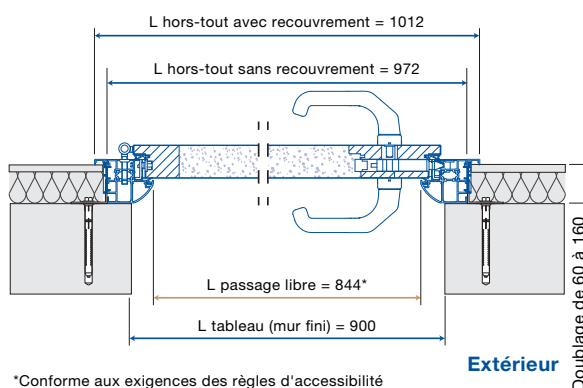
COUPE EN LARGEUR
