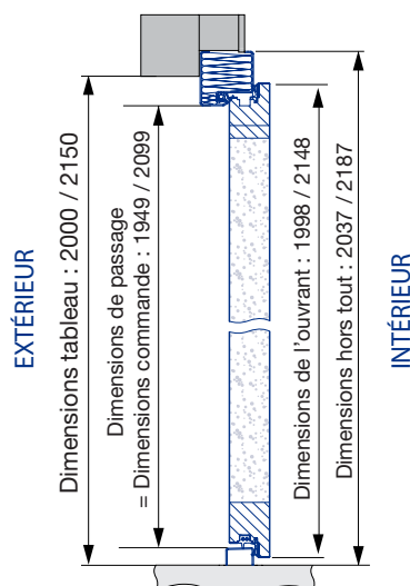
COUPE EN HAUTEUR
