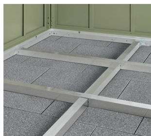
Ossature métallique pour planchers et plaque de sol en aluminium
