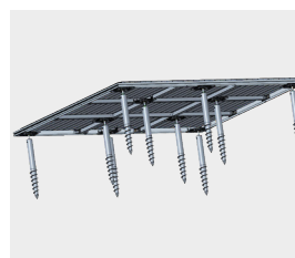
Fondation vissée réglable pour cadre et ossature métallique
